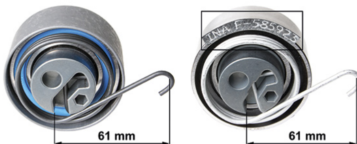
Рис. 1: 531 0535 20 – прежняя конструкция (слева), новая конструкция (справа)
