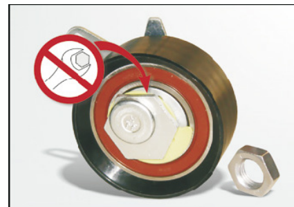
Рис. 2: Шестигранный элемент на задней стороне натяжителя не имеет функционального назначения.
