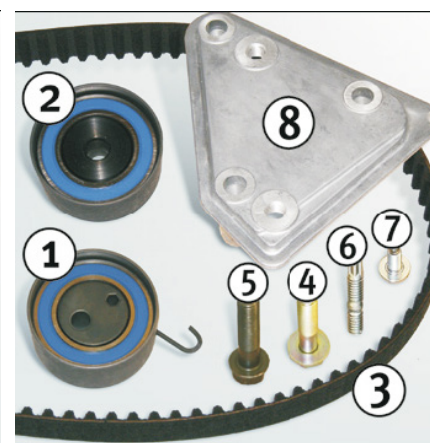
Рис. 2: Состав упаковки: 530 0492 10
