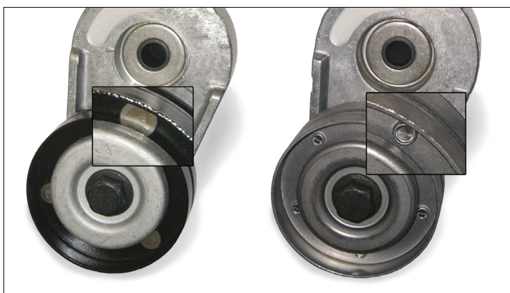
Рисунок 1: Детальное изображение роликов предыдущей (слева) и новой (справа) конструкции
