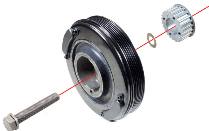
Рисунок 1: Комплект ременного привода состоит из демпфера крутильных колебаний коленчатого вала, крепежного болта и шайбы с алмазным напылением.
