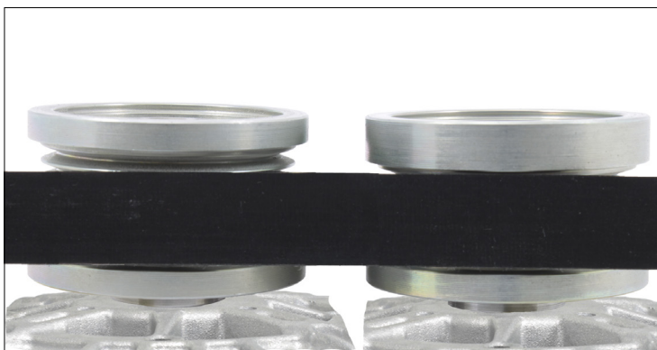
Рисунок 1: Слева шкив генератора с обгонной муфтой с 6 канавками, артикульный номер 535 0202 10 – шкив генератора с обгонной муфтой с 5 пазами
